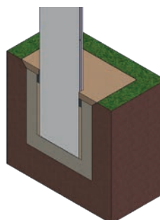
Avec massif en scellement direct
