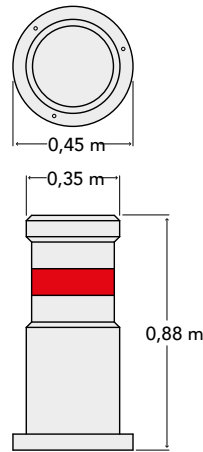
Balise Vigilo 350 Poids 57 kg
