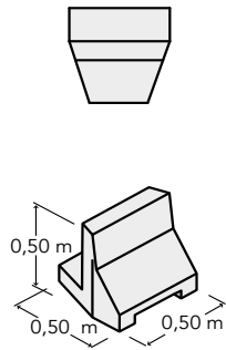
Élément droit court PL 2
