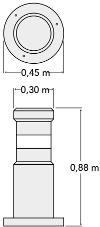
Balise Vigilo 300 Poids 48 kg
