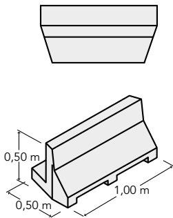
Élément droit long PL 1
