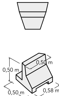
Élément pour courbe PL 3
