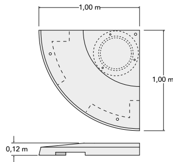
Plateau Vigilo Poids 57 kg
