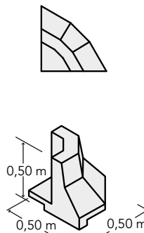
Élément d'angle PL 4
