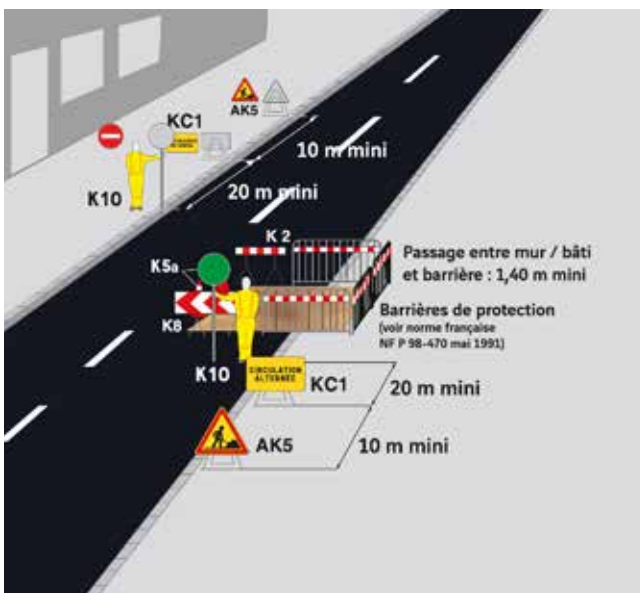
ALTERNAT PAR PIQUETS EN VOIE URBAINE
